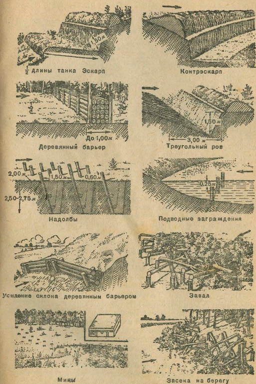
Рис. 17. Наиболее употребительные противотанковые препятствия
